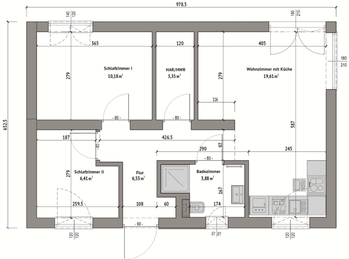
Grundriss DV-150-A
