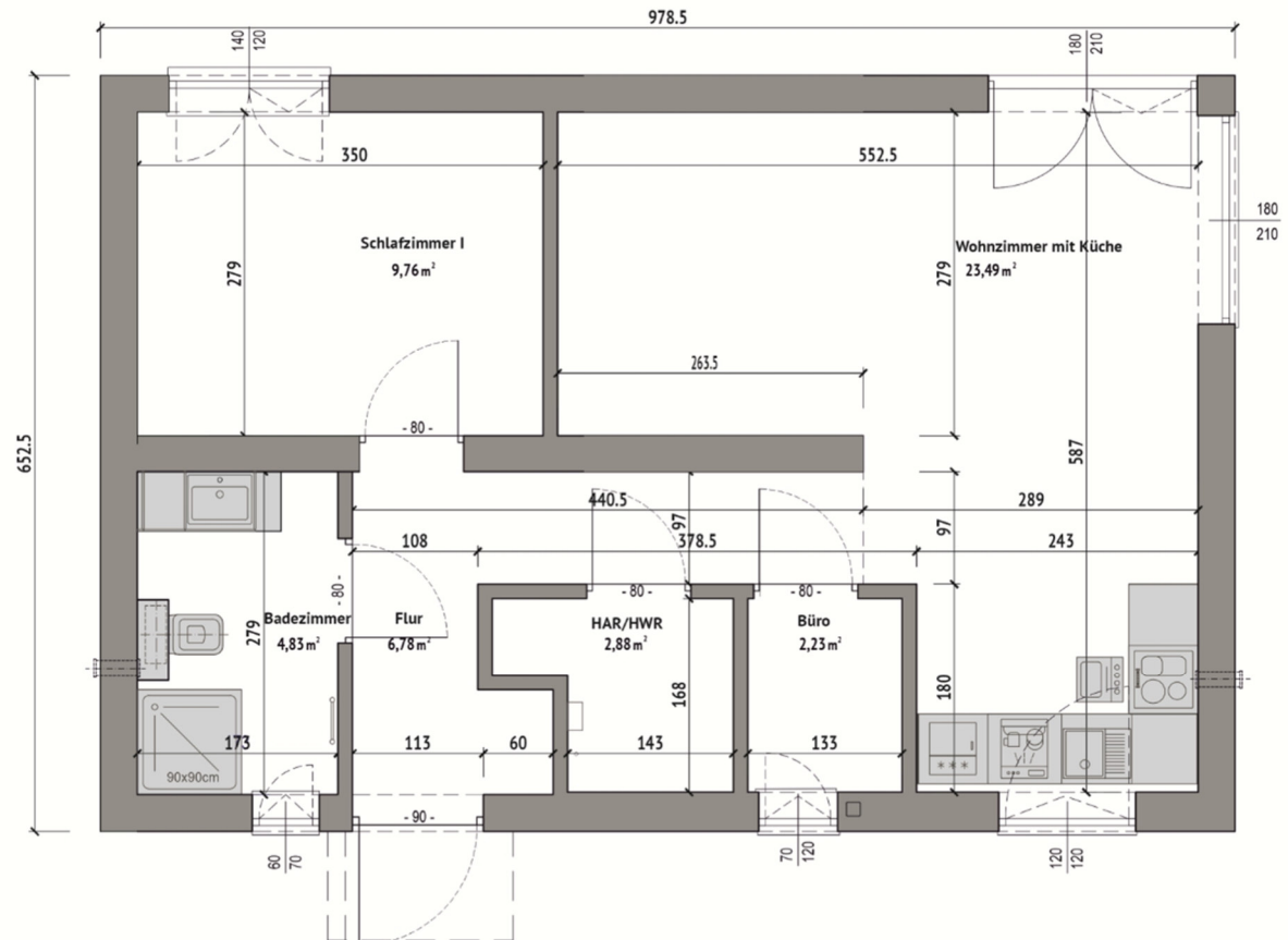
Grundriss DV-150-B
