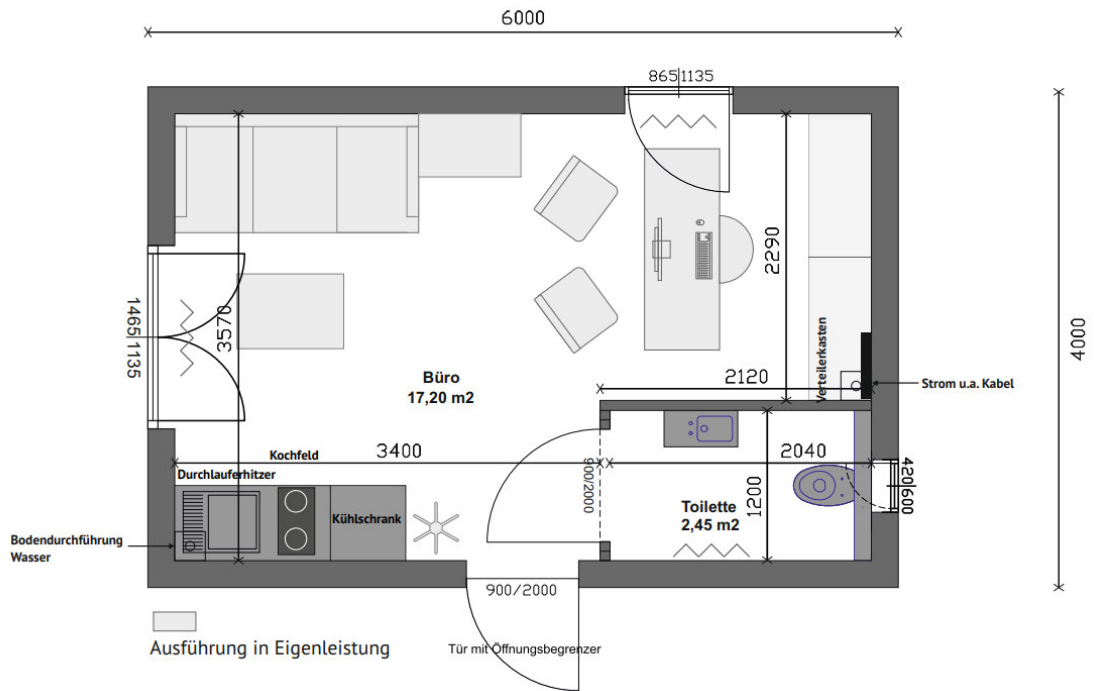
Technische Zeichnung. Möblierung zur Veranschaulichung
