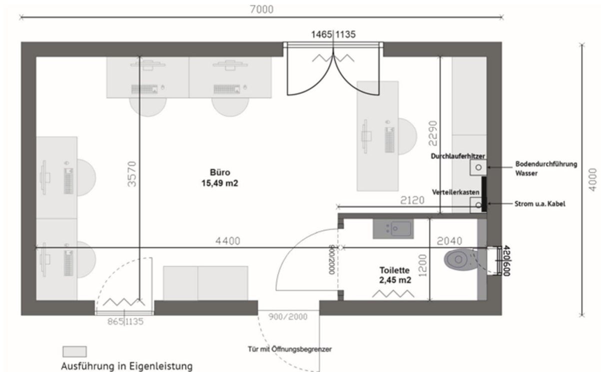
Technische Zeichnung. Möblierung zur Veranschaulichung
