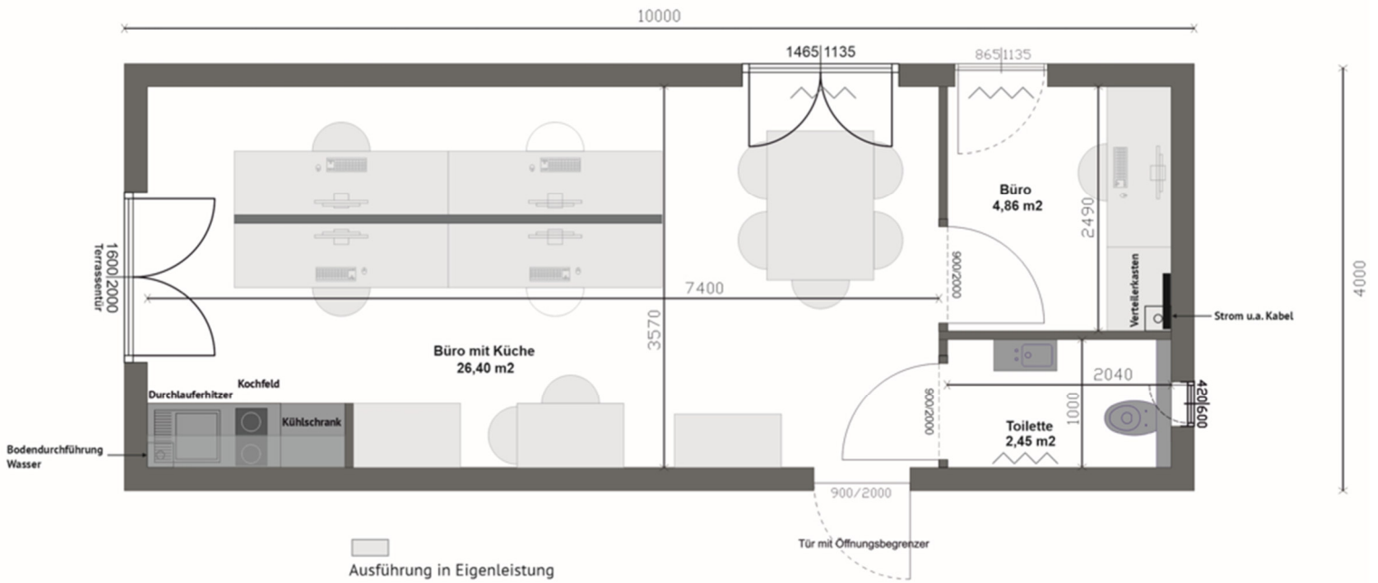
Technische Zeichnung. Möblierung zur Veranschaulichung
