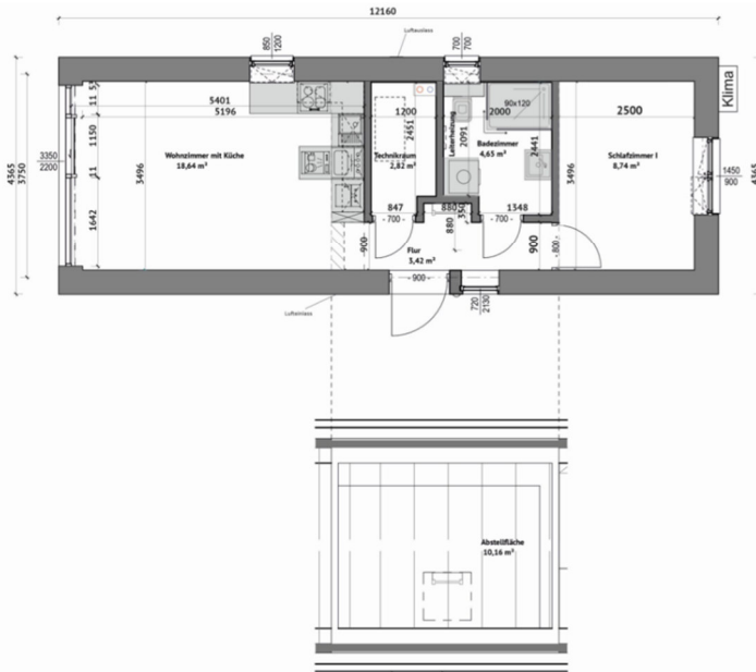
Technische Zeichnung. Möblierung zur Veranschaulichung
