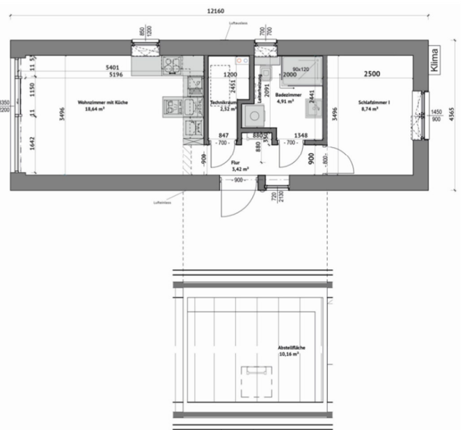
Technische Zeichnung. Möblierung zur Veranschaulichung
