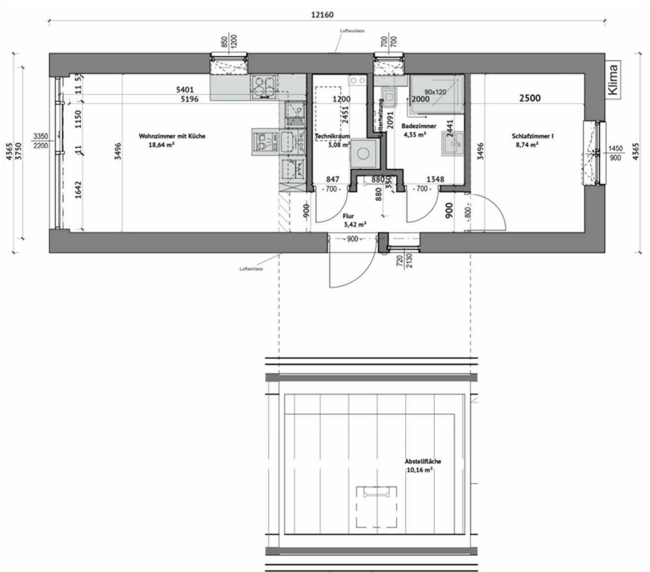
Technische Zeichnung. Möblierung zur Veranschaulichung
