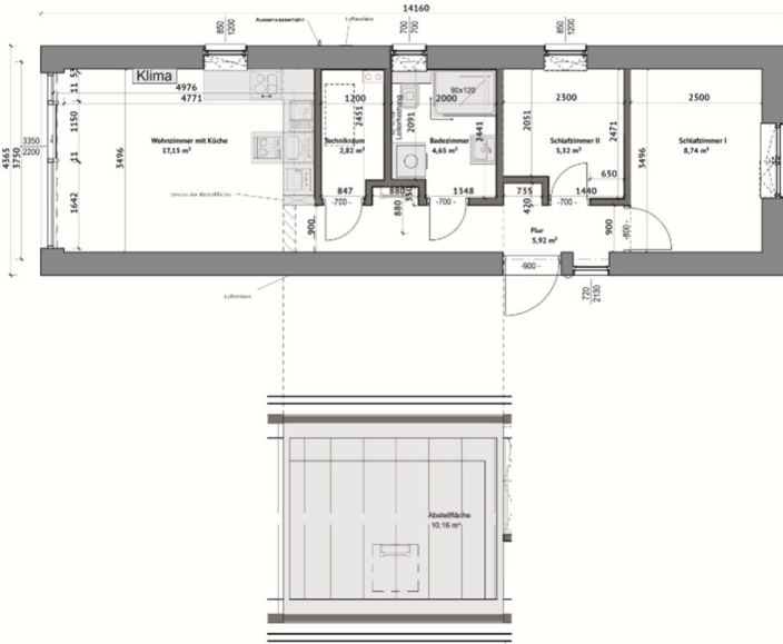
Technische Zeichnung. Möblierung zur Veranschaulichung
