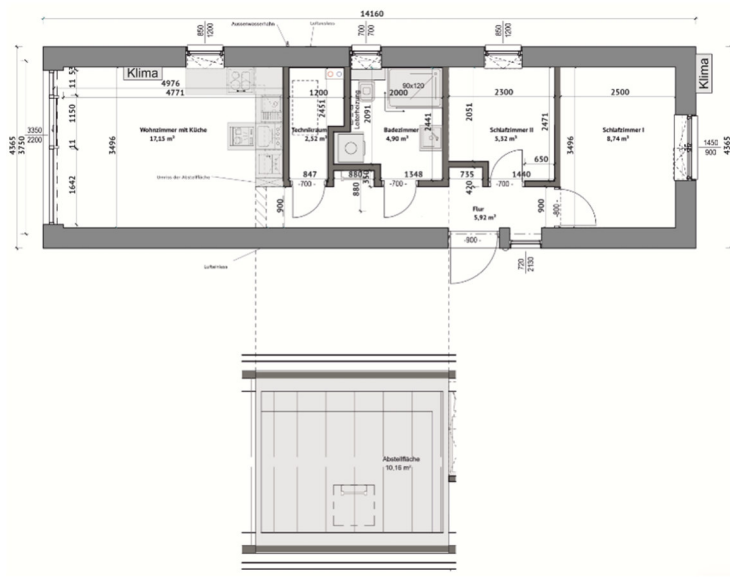
Technische Zeichnung. Möblierung zur Veranschaulichung
