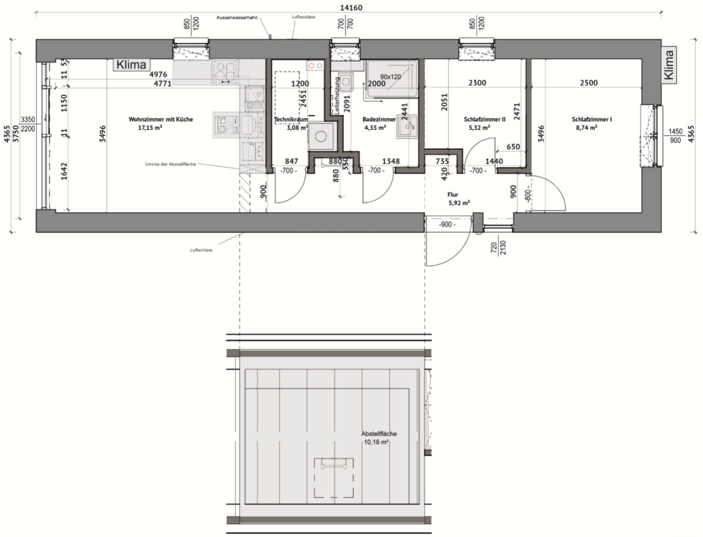
Technische Zeichnung. Möblierung zur Veranschaulichung
