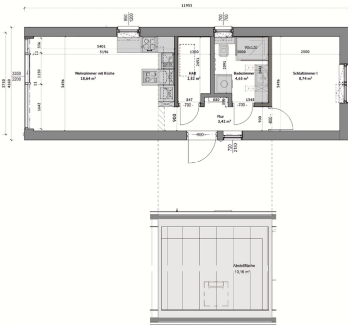
Technische Zeichnung. Möblierung zur Veranschaulichung
