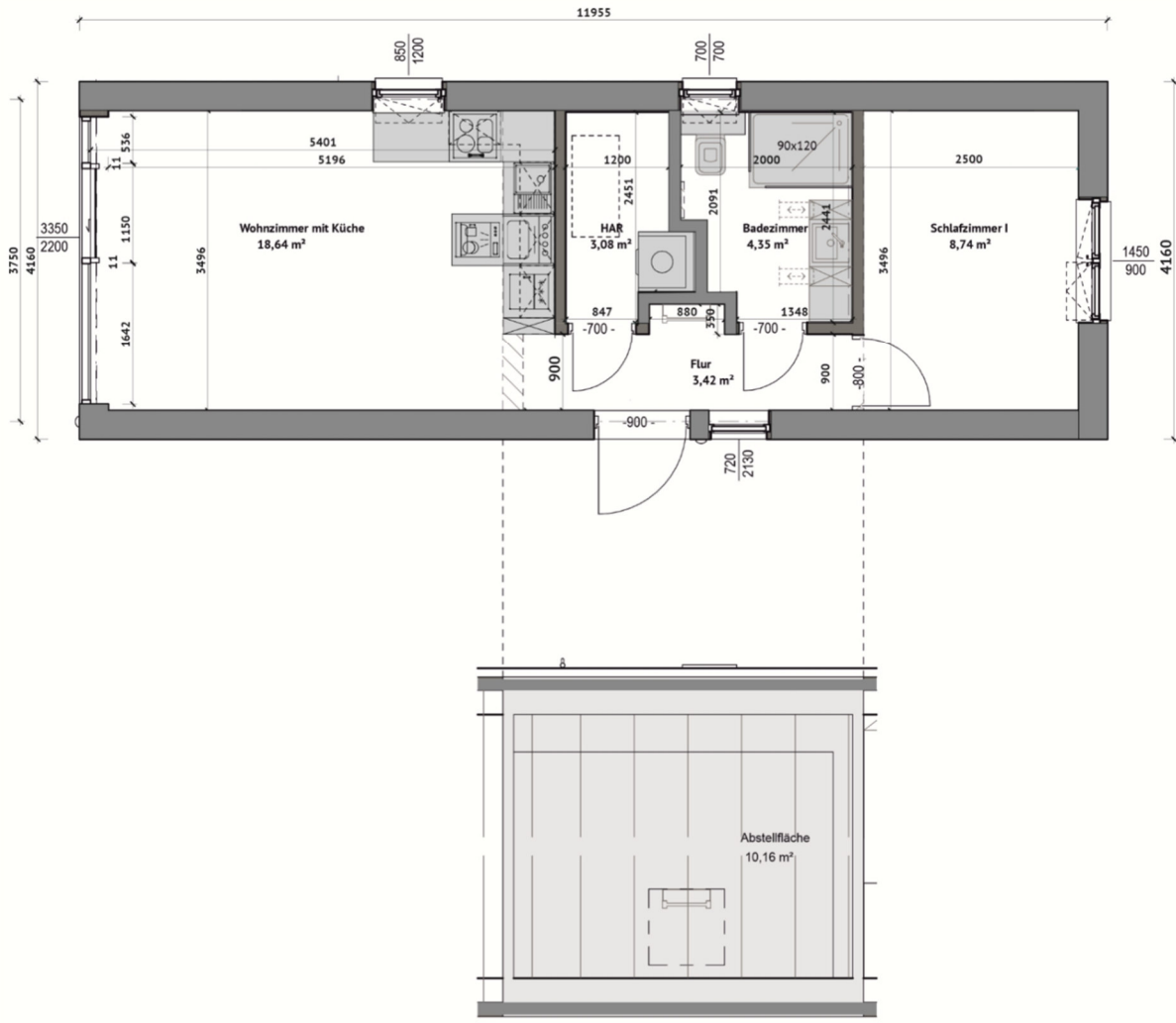
Technische Zeichnung. Möblierung zur Veranschaulichung
