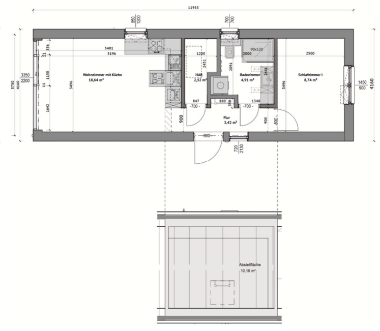
Technische Zeichnung. Möblierung zur Veranschaulichung
