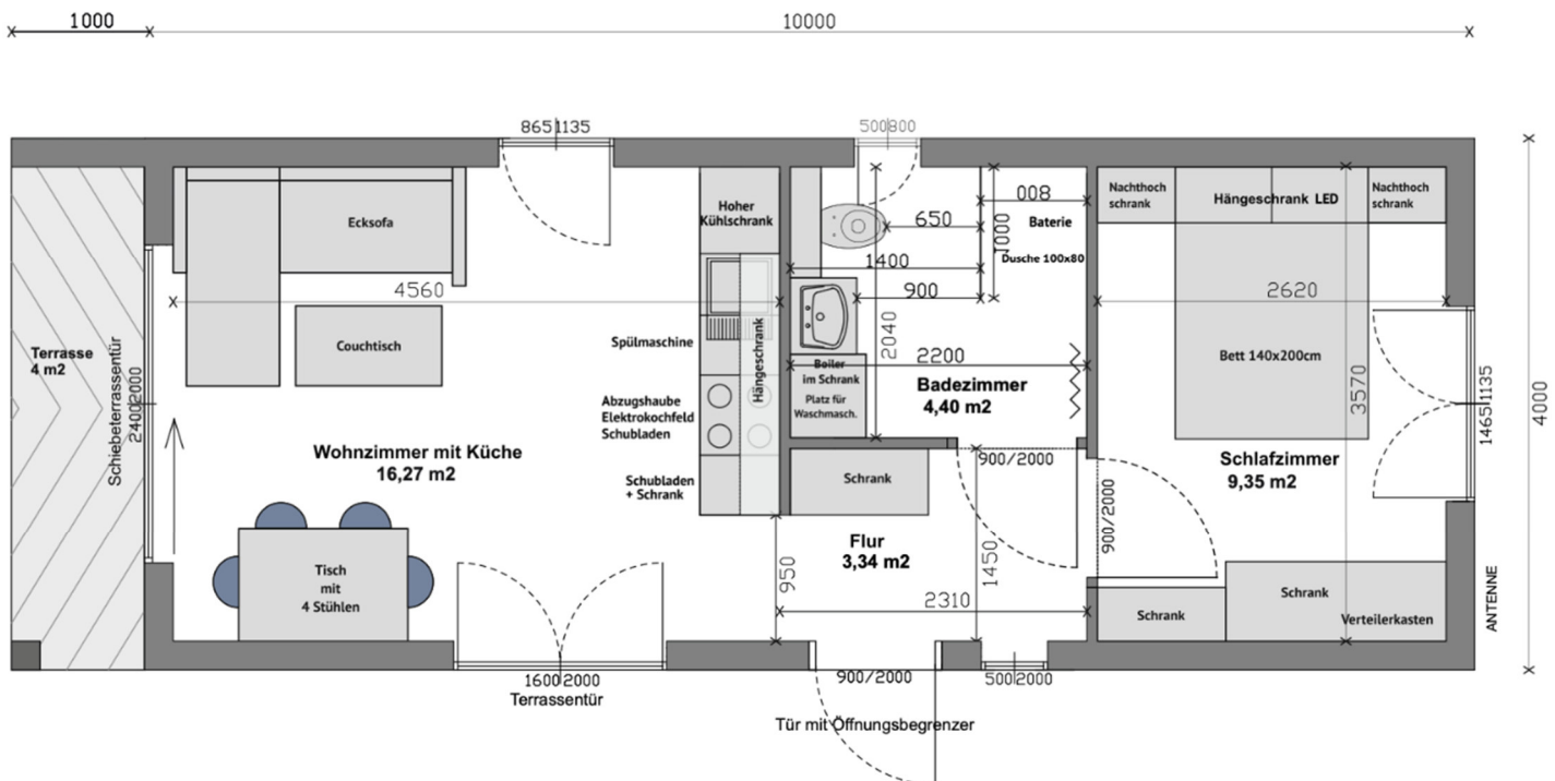
Technische Zeichnung. Möblierung zur Veranschaulichung
