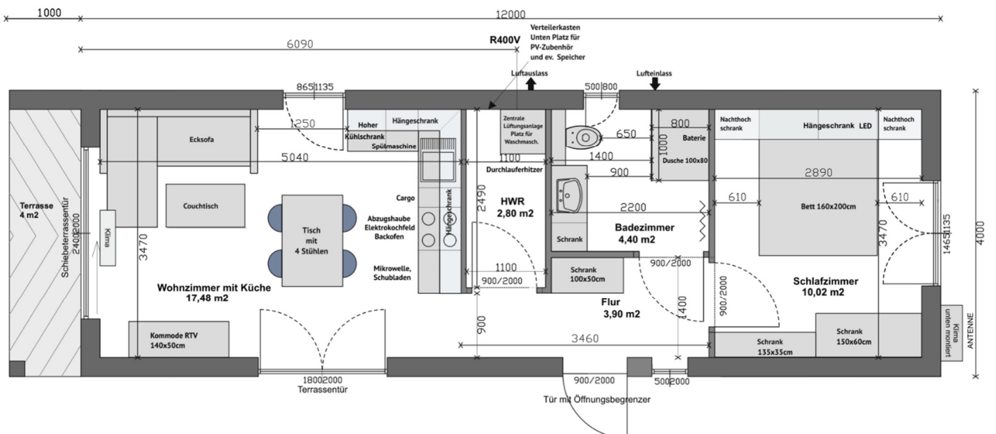
Technische Zeichnung. Möblierung zur Veranschaulichung
