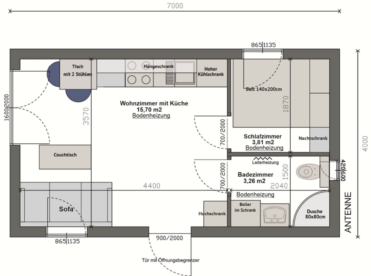
Technische Zeichnung. Möblierung zur Veranschaulichung
