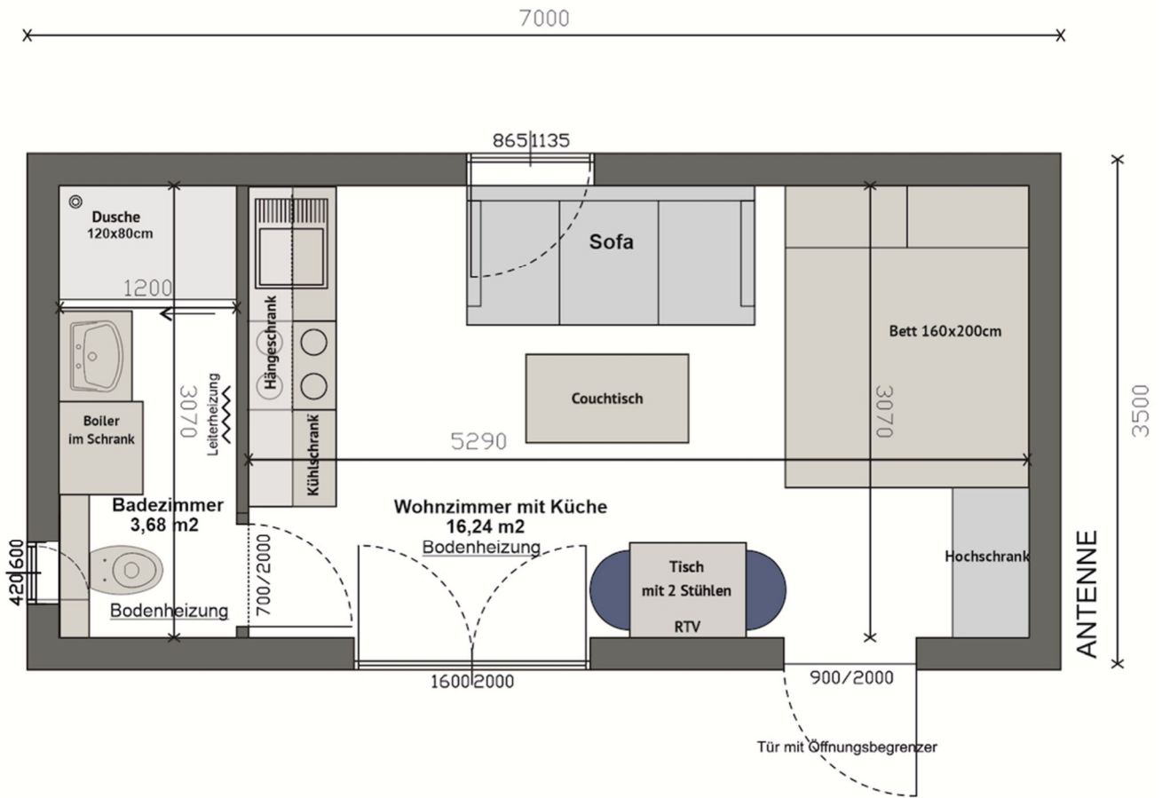
Technische Zeichnung. Möblierung zur Veranschaulichung
