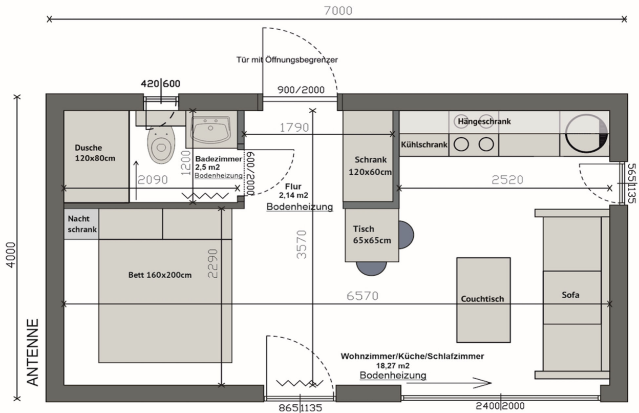
Technische Zeichnung. Möblierung zur Veranschaulichung
