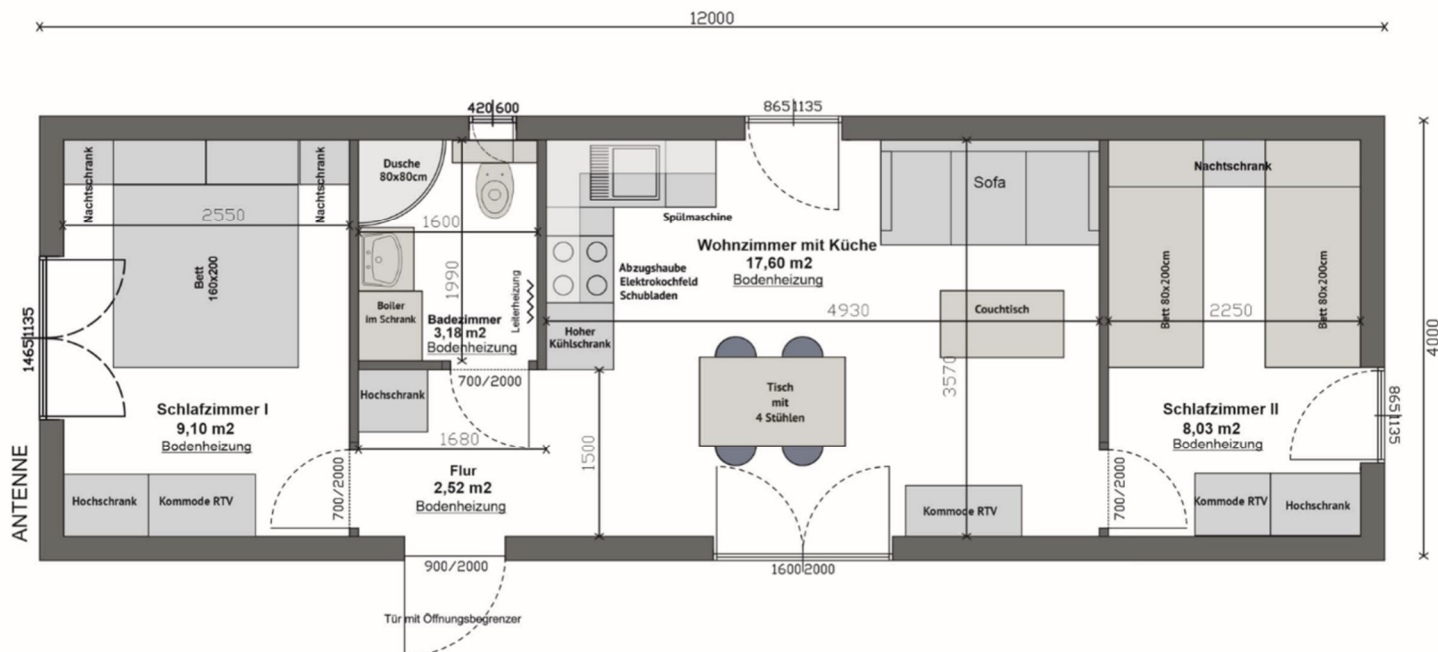
Grundriss MV48-4-A
